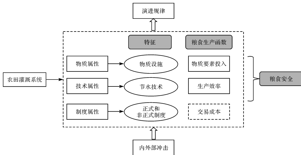
图1 农田灌溉系统对粮食安全的作用机制分析 个角度进行概括。
