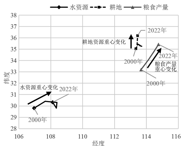
图1 2000—2022年粮食产量与水-土资源重心变化
