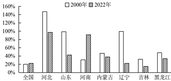
图2 2000年、2022年北方粮食主产区水资源开发指数 数据来源:2000年、2022年《中国水资源公报》。
