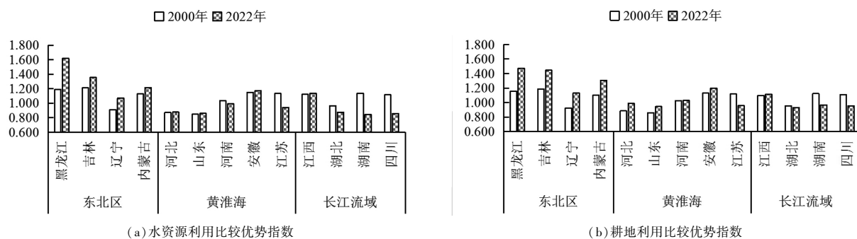
图3 2000年和2022年粮食主产区各省(区)水-土资源利用比较优势指数
